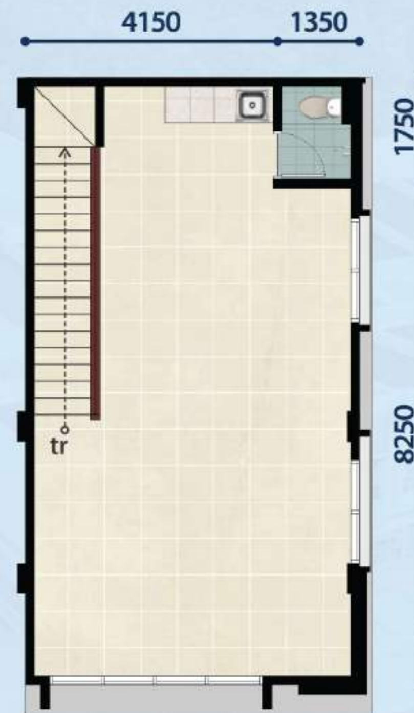
LANTAI 2
