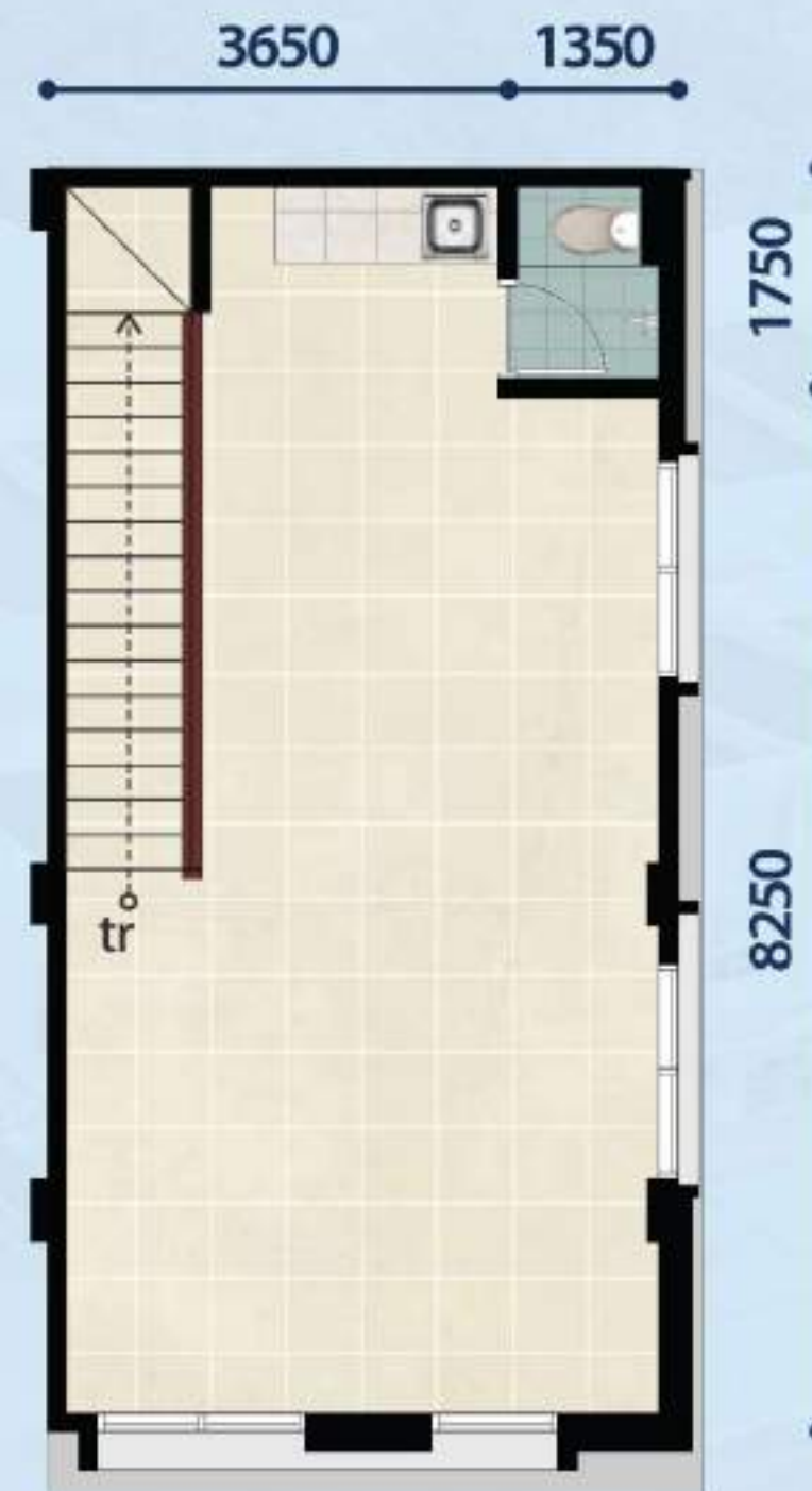
LANTAI 2
